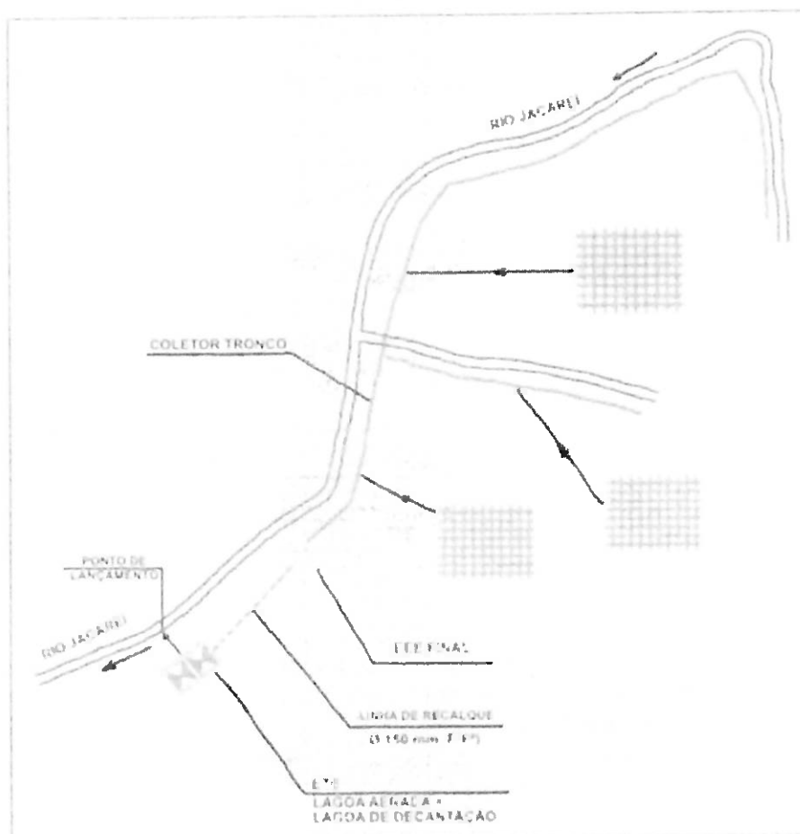
Figura 3 – Sistema de Esgotamento Sanitário da Sede do Município
